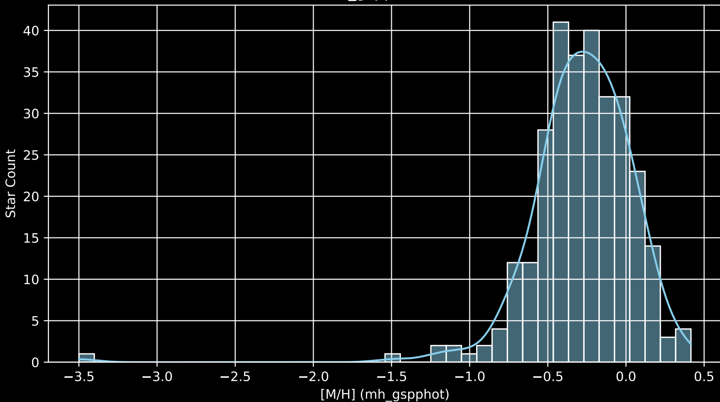
GALAH DR4 Field: [236] [M/H] (mh_gspphot) (n= 291)
