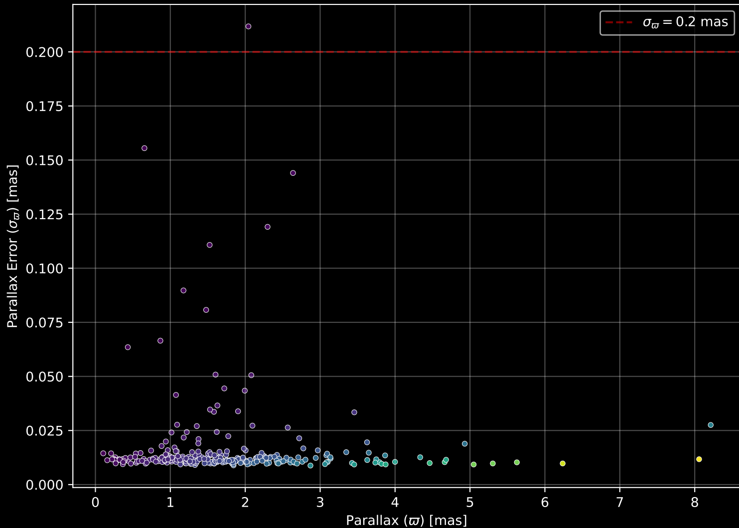
GALAH DR4 Field: [236] Parallax Quality (n= 294)
