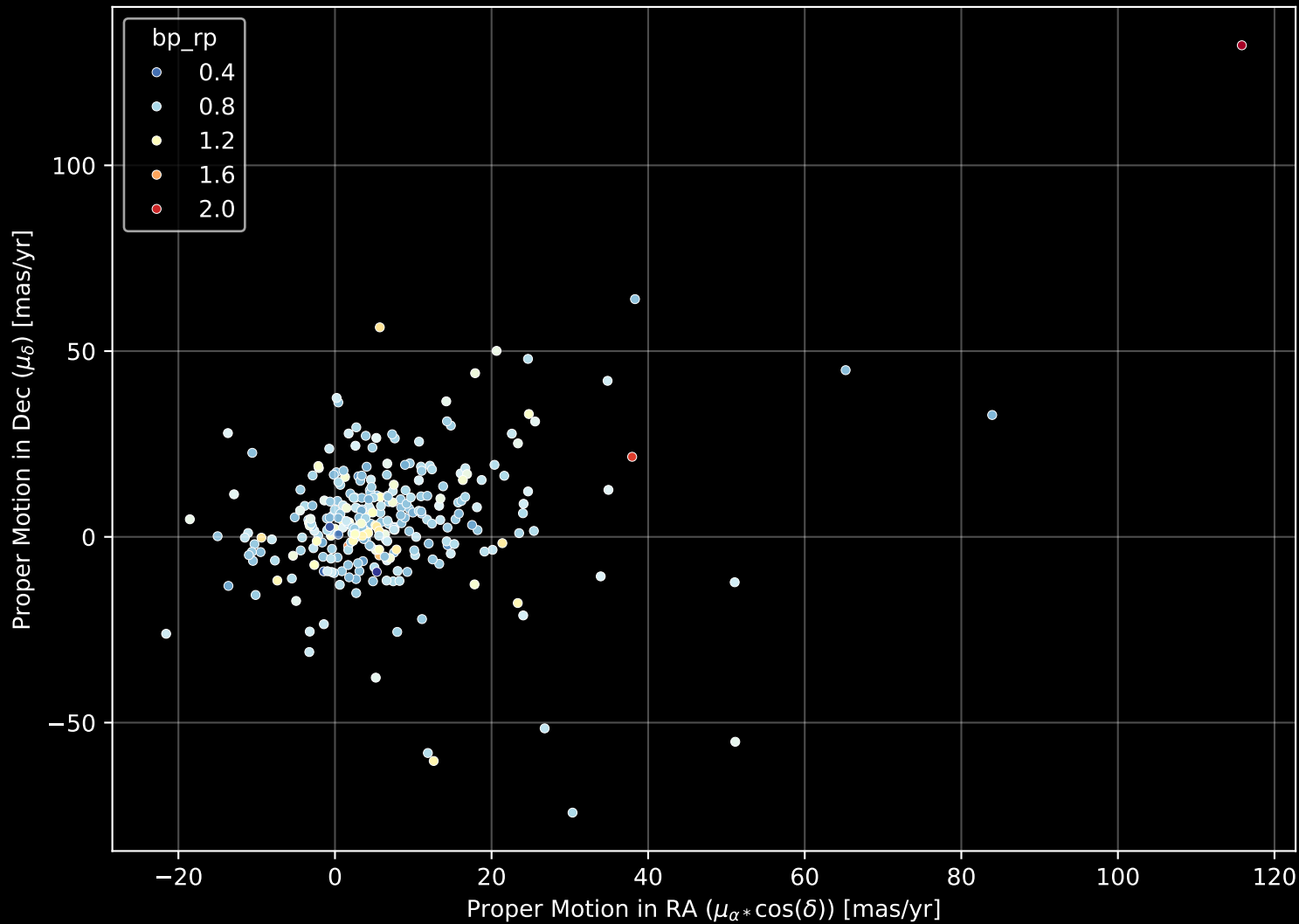
GALAH DR4 Field: [236] Proper Motion Diagram (n= 294)
