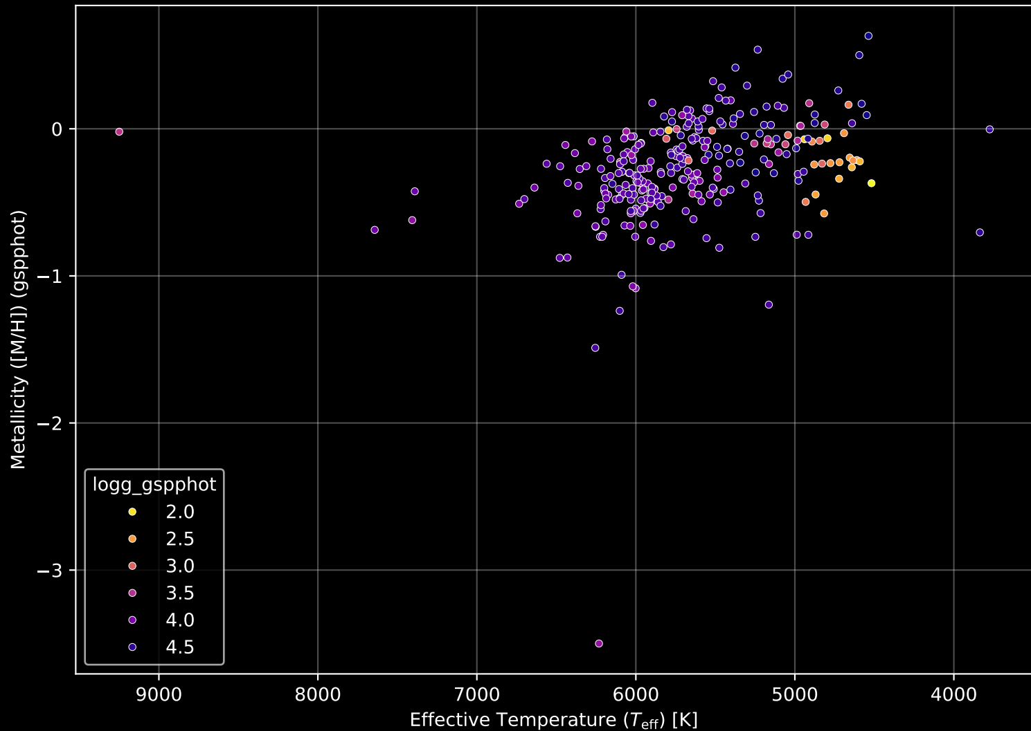
GALAH DR4 Field: [236] Stellar Population Parameters (n= 294)
